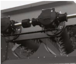
Graças à opção de inverter hidráulicamente os rotores convenientemente a partir da cabina, os bloqueios podem ser facilmente e idealmente limpos.
