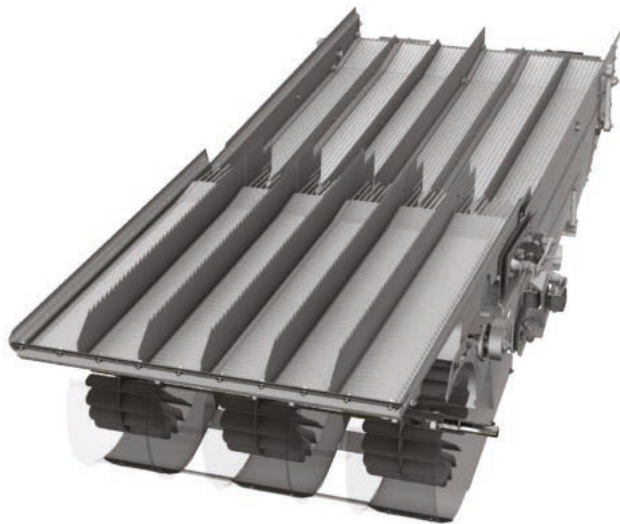
As 6 barras centrais medem 150 mm de altura para uma insensibilidade de inclinação de até 15 graus. Sensores de perda no final da sapata ajudam a ajustar a máquina para a melhor configuração possível.
